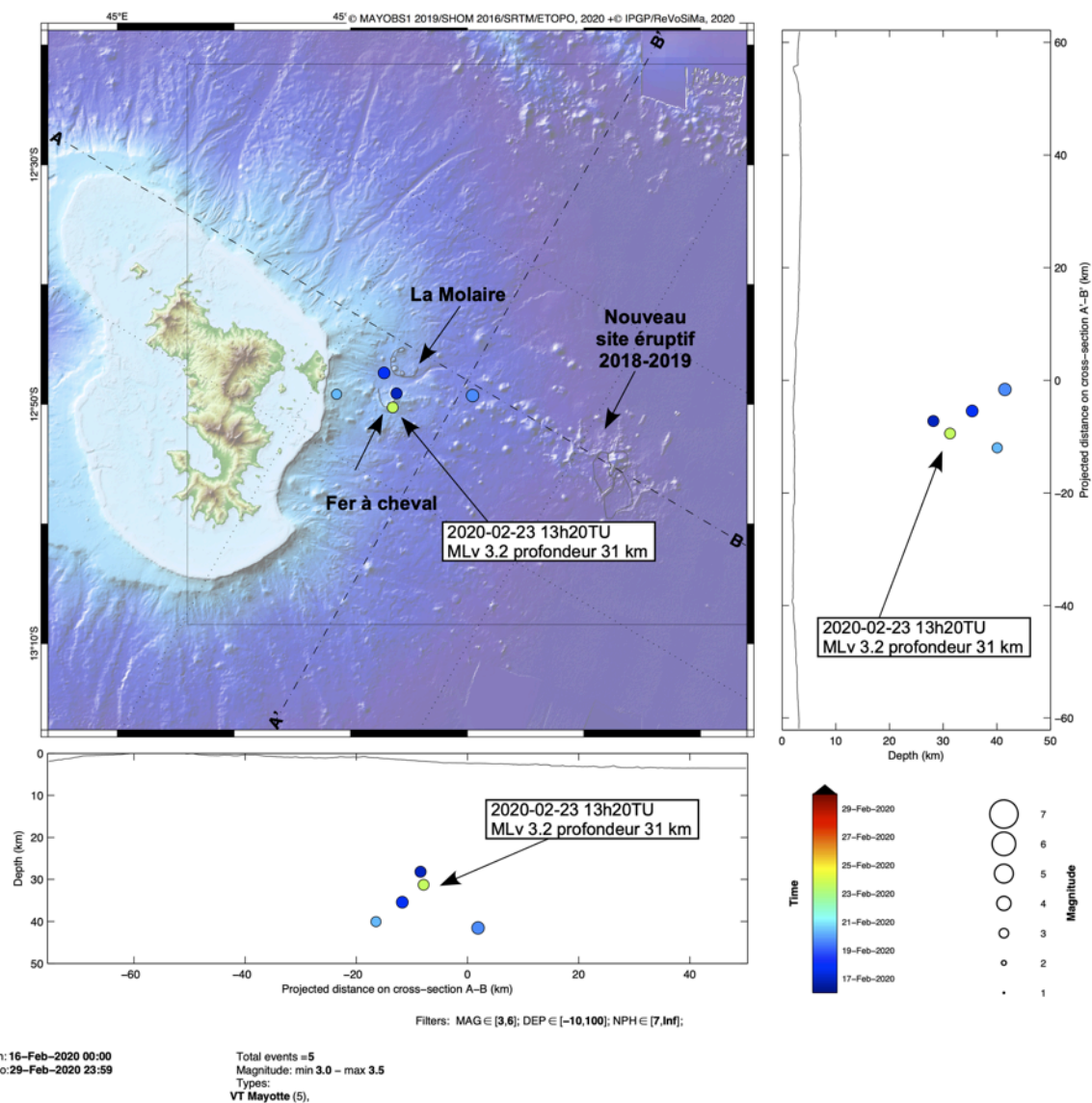
Figure 1b : Carte de localisation des épicentres ( \pm 5 km) des séismes volcano-tectoniques (VT) de magnitude M \geq 3 entre le 16 et le 29 février 2020 enregistrés avec les réseaux sismiques à terre (IPGP-IFREMER-CNRS-BRGM-BCSF-RéNaSS, IPGS). Sont aussi représentées une projection des hypocentres des séismes le long de coupes transverses et axiales le long de la ride montrant la localisation estimée en profondeur (la précision varie entre +5 km et +15 km) des séismes en fonction de la magnitude (taille des symboles) et de la date (échelle temporelle de couleur). Les structures volcaniques de la zone dite de « La Molaire », du « Fer à cheval » sont indiquées en grisé tout comme les coulées de lave du site éruptif actuel. De nombreux points de sortie de panaches de fluides dans la colonne d'eau ont été identifiés dans la structure du Fer à cheval avec une signature géochimique magmatique (voire section Géochimie des fluides). MNT d'après Feuillet 2019 et Shom 2016. (© OVPF-IPGP, BRGM, IFREMER, CNRS, BCSF-RéNaSS, IPGS / REVOSIMA).
