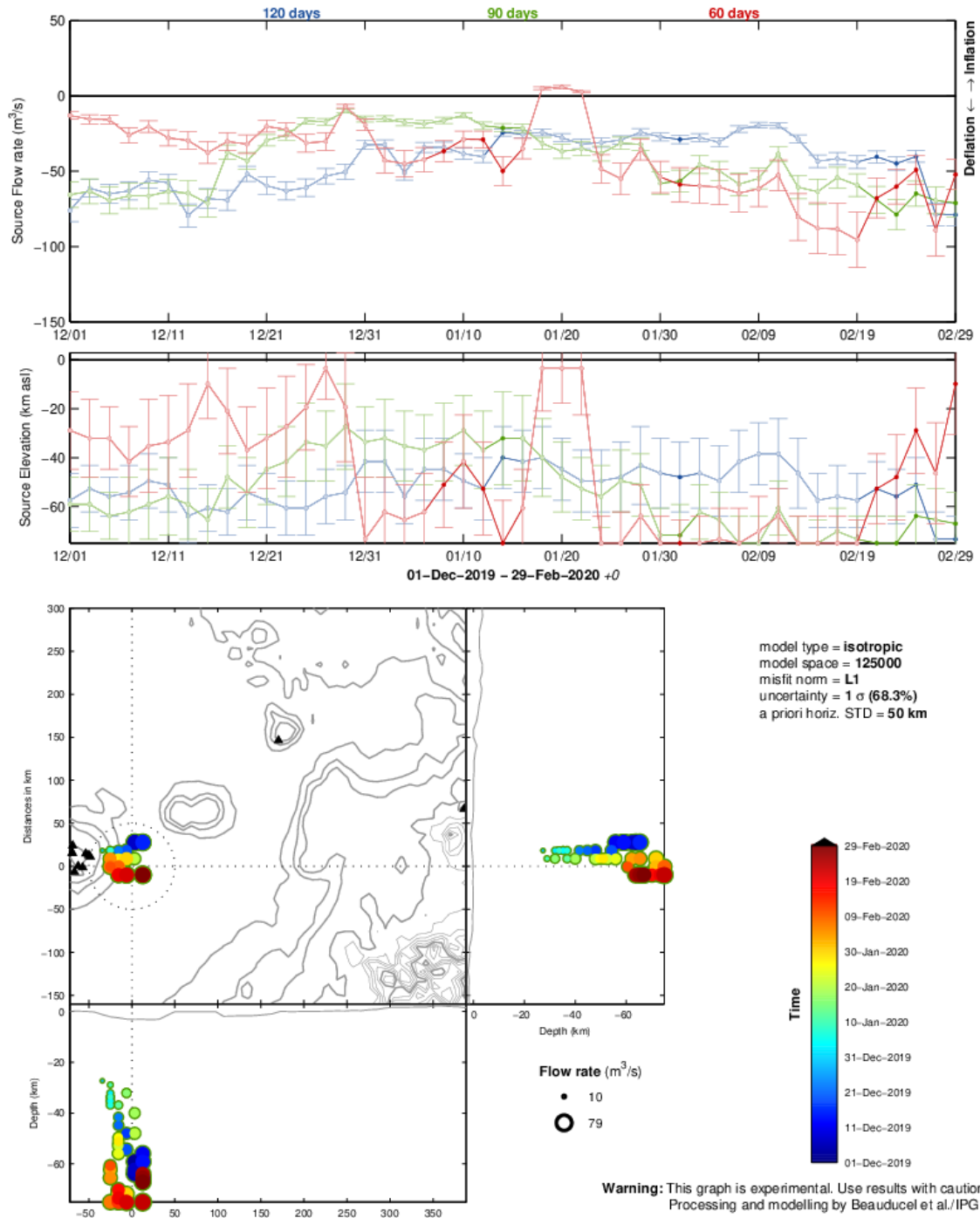
Figure 10 : Évolution spatio-temporelle du meilleur modèle de la source des déformations sur les trois derniers mois. Attention ce graphique ne prend pas en considération les incertitudes du modèle. Chaque point du graphe correspond au résultat d'une modélisation de la source prédominante calculée à partir des données GPS sur une période intégrée de 60 jours (rouge), 90 jours (vert) ou 120 jours (bleu). Le graphe supérieur indique le débit magmatique estimé (en mètres cube par seconde). Le graphe intermédiaire indique la profondeur de la source (en km sous le niveau de la mer). Les barres d'erreur indiquent l'écart de l'incertitude sur les paramètres à 68% de probabilité. Le graphe inférieur représente les projections horizontale (vue du dessus) et verticale (vues du sud et de l'est) des sources, la taille de chaque marqueur correspondant au débit magmatique ("Flow rate"), et la couleur à la date la plus récente des données utilisées pour chaque modèle (bleu foncé = 1 décembre 2019, rouge foncé = 29 février 2020). Ne sont représentés que les sources considérant une période intégrée de 90 jours. A noter que les positions de source et les valeurs de flux sur les derniers quinze jours sont à interpréter avec précaution car issues de calculs ne prenant pas en considération les orbites finales des satellites. Modélisations réalisées par F. Beauducel (IPGP/IRD) et OVPF-IPGP (©REVOSIMA).
