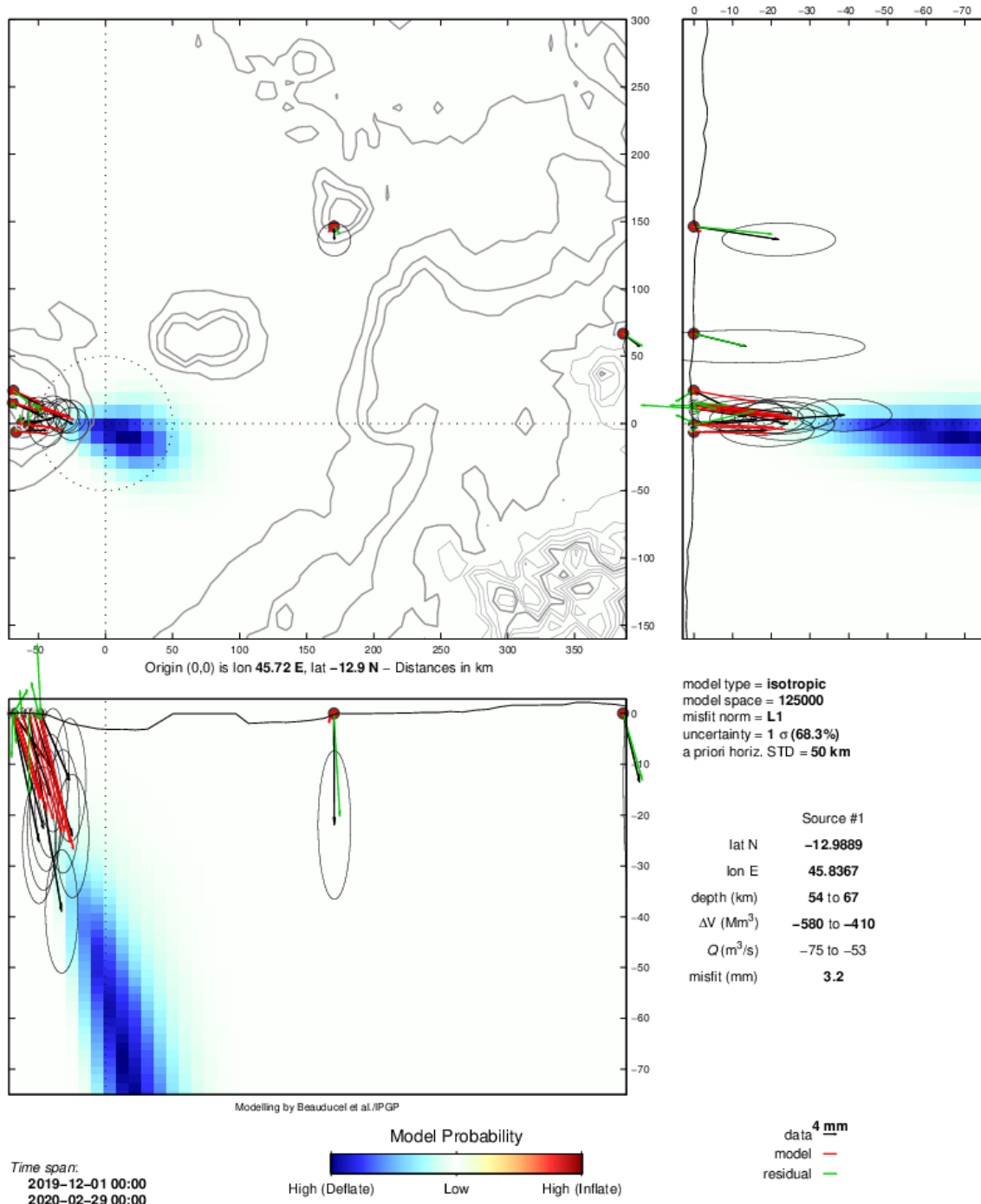
Figure 9 : Localisation de la source modélisée (meilleur modèle issu d'une modélisation de type isotrope point source) potentiellement à l'origine des déplacements enregistrés, au cours de la période : 1 décembre 2019– 29 février 2020, sur les stations GPS de Mayotte, Grande Glorieuse et DSUA (Madagascar). Les vecteurs en noirs représentent les données observées, les vecteurs en rouge représentent les données modélisées, et les vecteurs en vert représentent les résidus du signal qui n'ont pas pu être modélisés. L'échelle de couleur donne la probabilité en % de la localisation d'une source en déflation (dégradé de couleurs froides, bleus) ou en inflation (dégradé de couleurs chaudes, jaune-rouge) en latitude-longitude et en profondeur selon une représentation cartographique et en coupes verticales orientées est-ouest et nord-sud. Le modèle permet d'estimer la variation de volume de la source, en millions de m 3 (Mm 3 ) et son incertitude, qui explique au mieux les signaux enregistrés. En faisant l'hypothèse que cette variation de volume traduit des transferts de magma dans la lithosphère, le modèle permet d'avoir une estimation préliminaire du flux en m 3 /s de magma associé à la déflation. Modélisations réalisées par F. Beauducel (IPGP/IRD) et OVFP-IPGP (©REVOSIMA).
